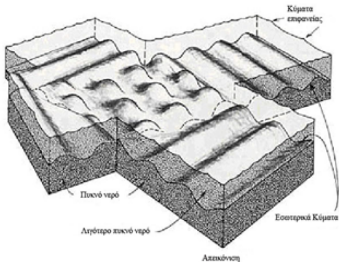
Εικόνα: Εσωτερικά κύματα στο σημείο επαφής δύο στρωμάτων νερού με διαφορετικές πυκνότητες. Το ένα είναι πυκνό (το κατώτερο), το άλλο είναι
