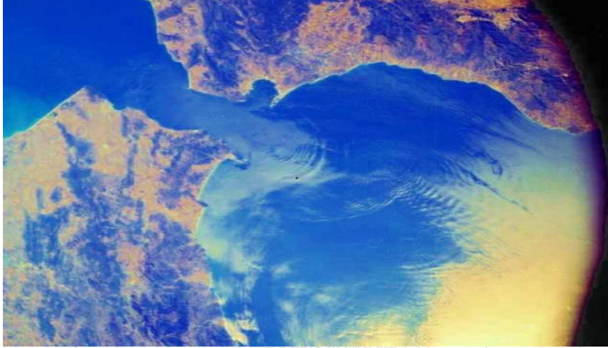
صورة مأخوذة بالأقمار الاصطناعية لمضيق جبل طارق، حيث تبين حدود مياه البحر الأبيض المتوسط الساخنة والمالحة عند دخولها في المحيط الأطلسي ذي المياه الباردة والأقل ملوحة.
