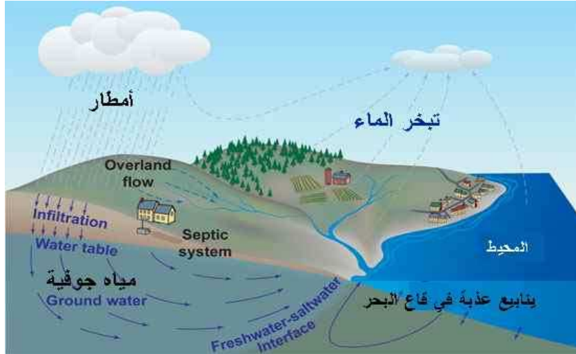
رسم يوضح دورة امتزاج الماء العذب بالماء المالح.
