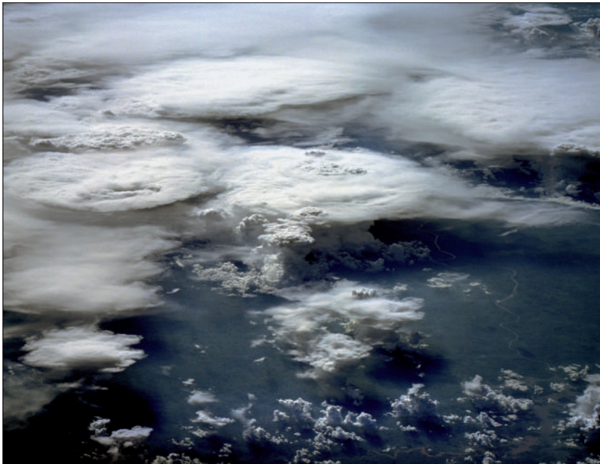
► Ett cumulonimbus-moln (bymoln eller åskmoln). Den här bilden har tagits av NASA satellit. Det ser ut som om en osynlig hand driver cumulusmolnen till konvergensområde.
