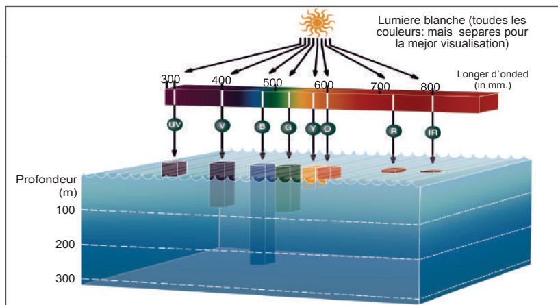
► Diagrammet visar djupet i havsvatten och ljusstrålar som tränger in i det. Eftersom rött ljus absorberas starkt har den ytlig penetrationsförmåga, och blått ljus har den djupaste penetrationsförmåga. (Applied Optics, 20 vol. (177) Smith, RC och KS Baker. 1981) Se även officiella NASA-s hemsida.
