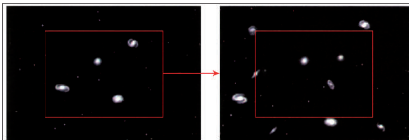
► Bilden visar att avstånden mellan galaxer (stjärnsystem) och galaxkroppar ökar hela tiden. Därför expanderar universum .
