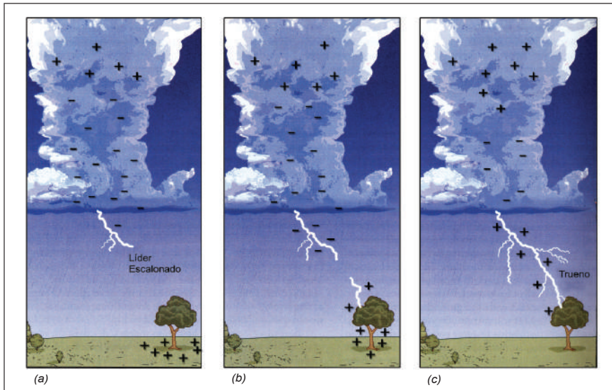
► Modell för sicksackblix. (a) Den negativa laddningen koncentrerad vid molnets botten blir tillräckligt stor för att övervinna luftens motstånd och utvecklar en "ledare" som pekar mot marken. (b) Ett uppåtriktat flöde av positiva laddningar från marken bildas vid upphöjd plats. (c) Det nedåtgående flödet av negativa laddningar möter det uppåtgående flödet av positiva laddningar och en stark elektrisk ström uppstår som i ett returslag bär de positiva laddningarna in i molnet.
