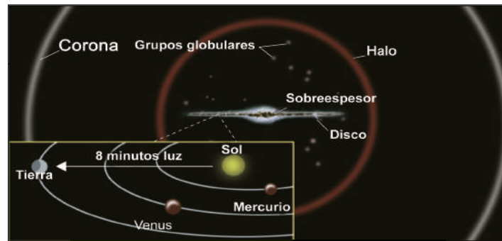
► Bilden visar galaxen och de olika planeterna.
