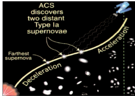
► Bilden visar att universum expanderar.
