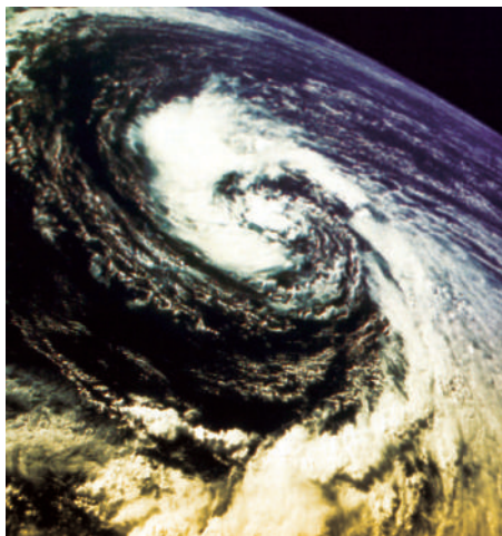
► En bild av atmosfären inklusive dess moln och vindar
