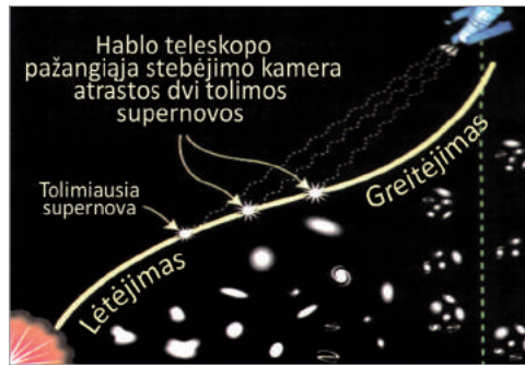
► Ši iliustracija vaizduoja Visatos plėtimąsi.
