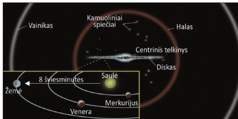
► Šiame paveikslėlyje pavaizduota mūsų galaktika ir planetos.
