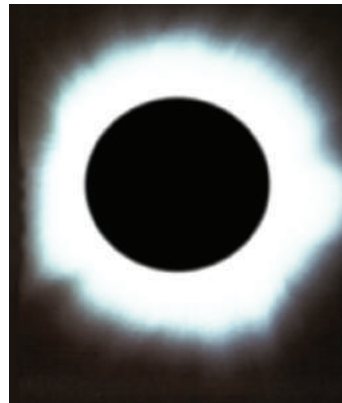
► Saulės užtemimas įrodo, kad Visata skendi tamsoje.
