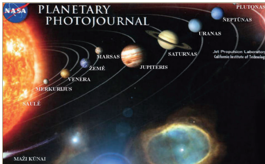
► Paveikslėlyje pavaizduota Saulės sistema.
