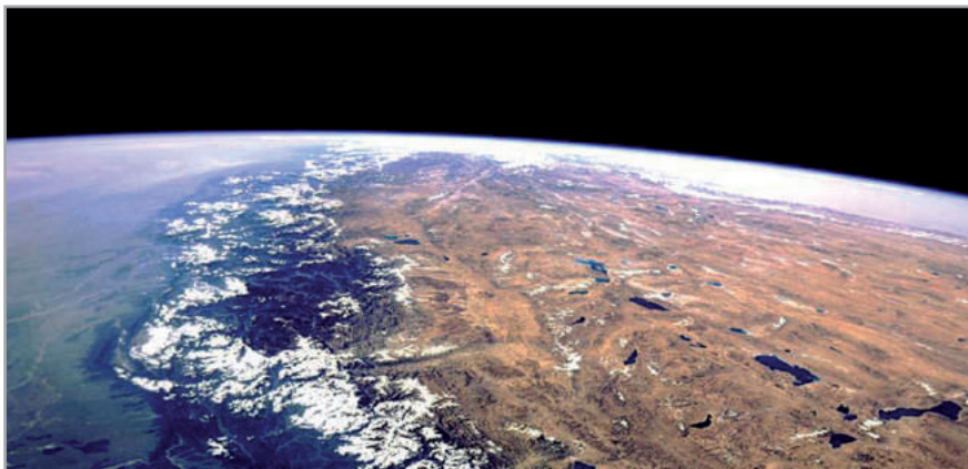
► Saulės apšviesta Žemė. Mums matoma tik nedidelė atmosferos dalis (iki 200 km aukščio) – visa kita skendi visiškoje tamsoje.
