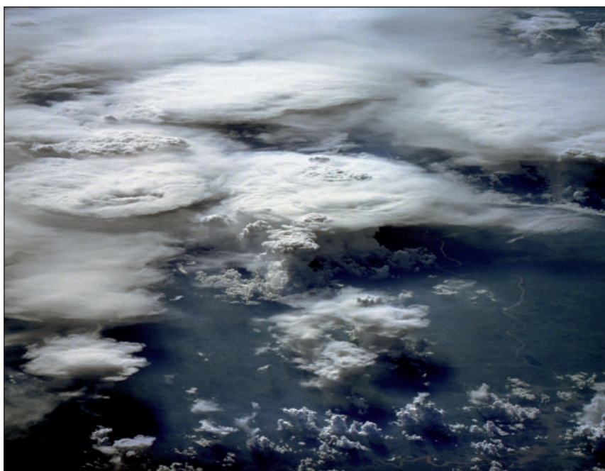
► Lietaus kamuoliniai debesis (lot. Cumulonimbus). Nufotografuota iš NASA palydovo. Nuotraukoje matome, kaip kamuoliniai debesis, tarsi juos gintų neregima ranka, renkasi tam tikroje vietoje.
