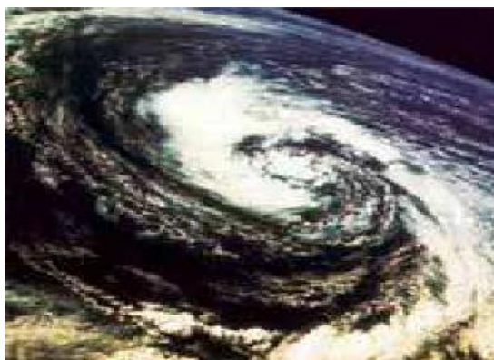
Atmosféra včetně oblak a větrů
