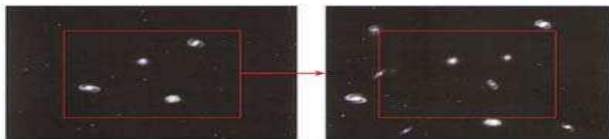
Tento obrázek ukazuje, že vzdálenost mezi galaxiemi či kupami galaxií se neustále zvětšuje a že vesmír se tedy rozpíná.
