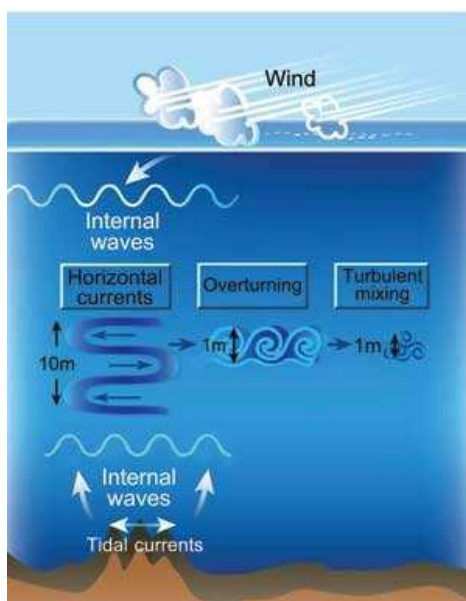
Vnitřní vlny a míchání vod v oceánu. (Oceanography, Chris Garrett. Více také na http://www.nature.com/nature/journal/v422/n6931/full/422477a.html )
