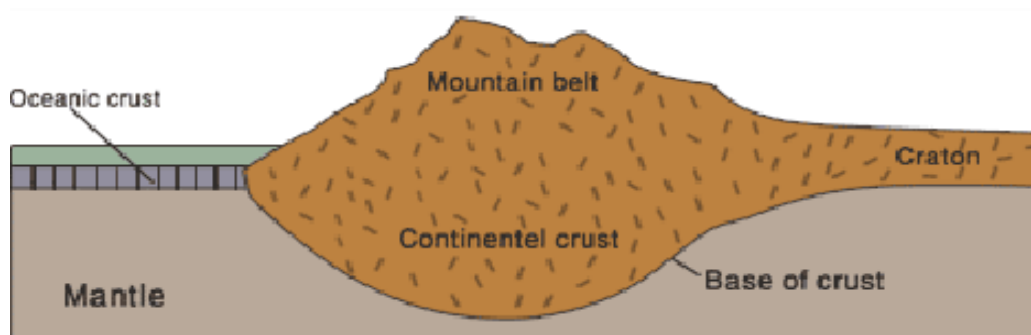
Obrázek znázorňuje „kořen“ hory. Některé tyto kořeny mohou zasahovat šedesát kilometrů hluboko do země.
