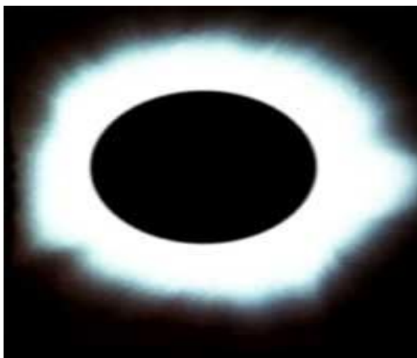
Toto je pohled na slunce během zatmění, který dokazuje, že ve vesmíru je tma.
