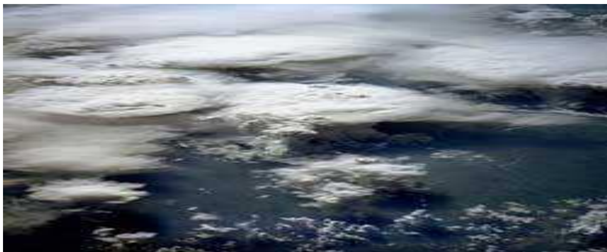
Oblak cumulonimbus, záběr pořízený satelitem NASA. Zdá se, jako by oblaka cumulus do zóny konvergence tlačila neviditelná ruka.
