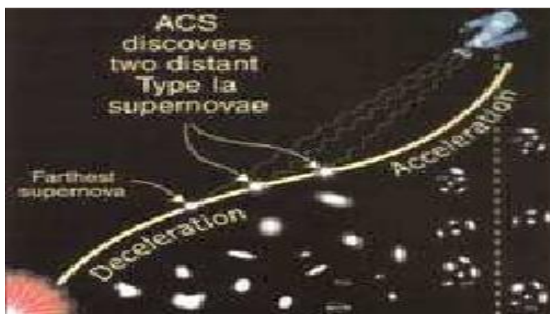
Tento obrázek znázorňuje, že se vesmír rozpíná.
