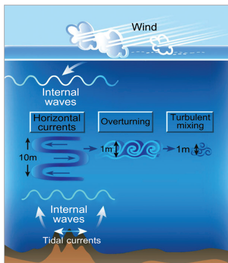
► A belső hullámok és az óceán keveredésének fokozatai. (Chris Garrett, Óceánográfia. Lásd még: http://www.nature.com/nature/journal/v422/n6931/full/422477a.html )
