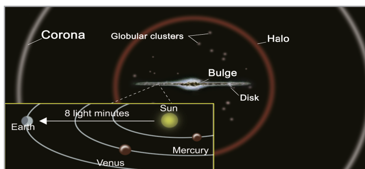
► Ez a fotó a Tejút galaxist mutatja és különböző bolygókat.
