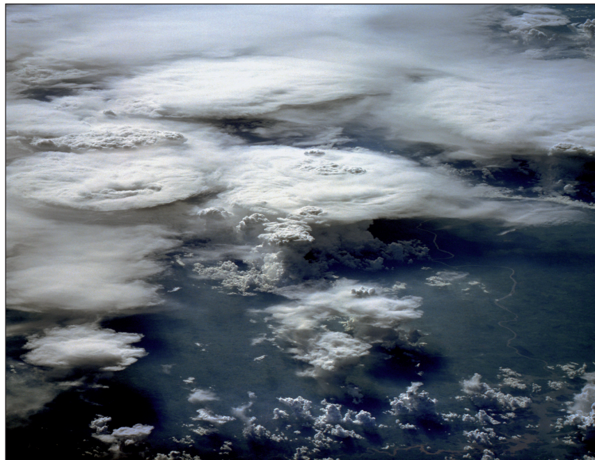
► Egy cumulonimbus felhő (viharfelhő). A képet a NASA műholdja készítette. Olyan, mintha egy láthatatlan kéz tolt volna a cumulus felhőket az összefutás helye felé.
