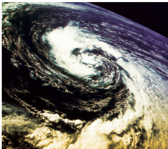
► A légkör képe, felhőkkel és szelekkel.
