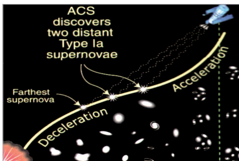
► Ez a kép azt mutatja, hogy az univerzum tágul.
