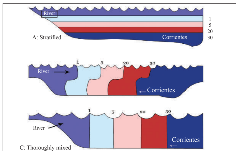
► Tři typy stratifikace salinity v pobřežních vodách
