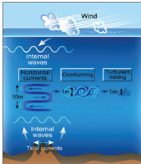
► Vnitřní vlny a míchání vod v oceánu. (Chris Garrett, Oceanography . Více také na http://www.nature.com/ )
