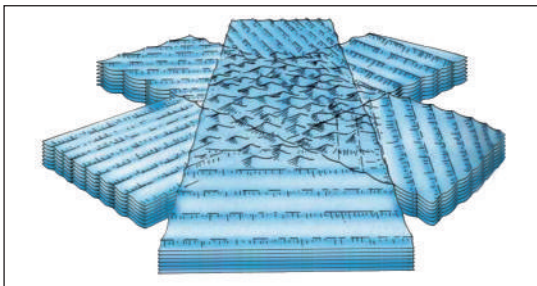
► Vnitřní vlny na rozhraní dvou vrstev vody o různých hustotách. Jedna (spodní) je hustá, druhá (horní) je méně hustá. (Gross, Oceanography , str. 204)
