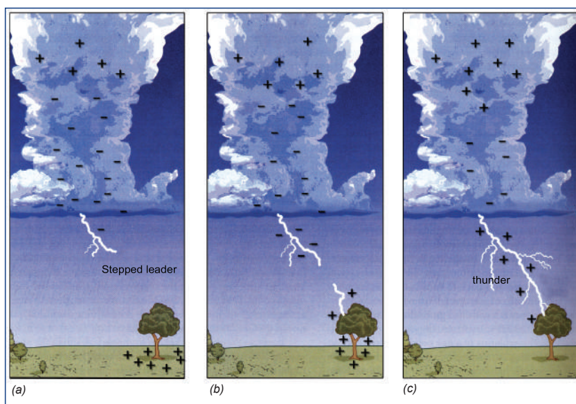
► Model rozvětveného blesku. (a) Záporný náboj koncentrovaný ve spodní části oblaku zesílí natolik, že jej už izolující vrstva vzduchu neudrží a vytvoří se vůdčí výboj blesku mířící k zemi. (b) Vstříčný výboj s kladným nábojem vychází nejčastěji z vyvýšených míst na zemi. (c) Dochází ke spojení záporně nabitého vůdčího a kladně nabitého vstříčného výboje a vzniká mohutný elektrický proud, tzv. hlavní výboj blesku, kterým všechny náboje v oblaku zaniknou.
