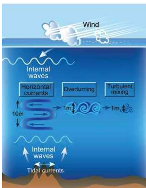
Vnútorne vlny a miešanie vôd v oceáne. (Oceanography, Chris Garrett. Viac tiež na http://www.nature.com/nature/journal/v422/n6931/full/422477a.html )
